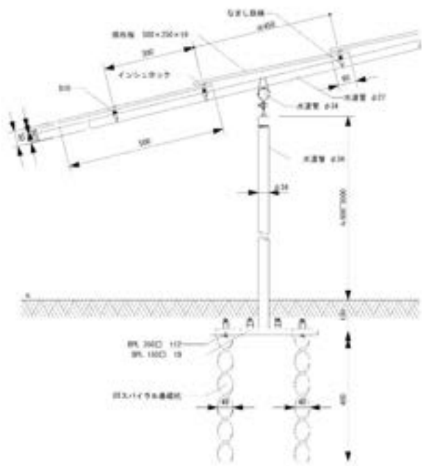
断面詳細図 S=1/10
